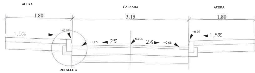
SECCION TIPO CALLE SAN ANTON. ESCALA: 1/50
