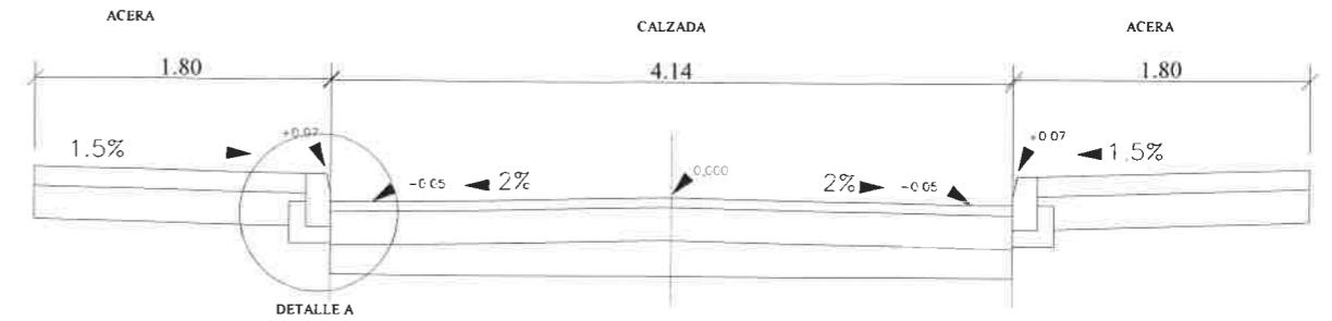
SECCION TIPO CALLE EL MOLINO. ESCALA: 1/50
